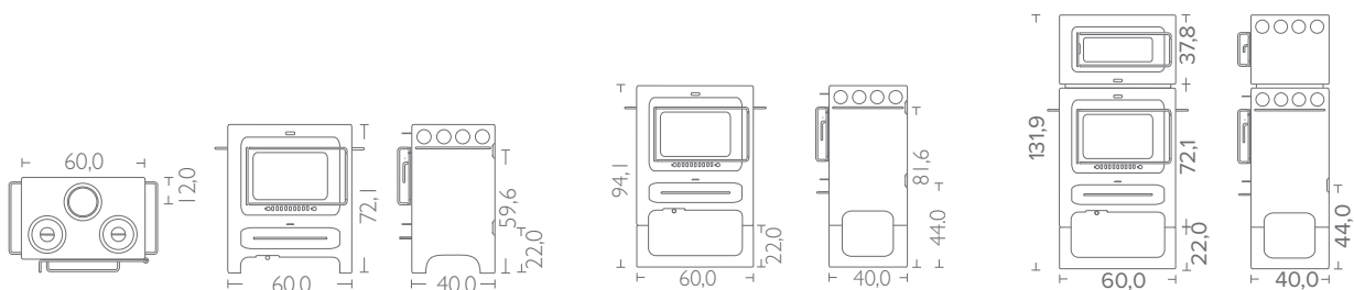
HWAM Classic 4 med bageovn og brændefag
