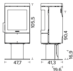
HWAM 3110c på piedestal Style greb (sort)
