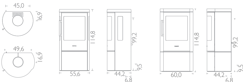
HWAM 3630c med sideglas
