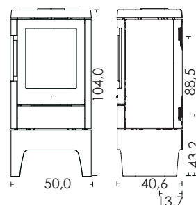
HWAM 4520m med høj sokkel
