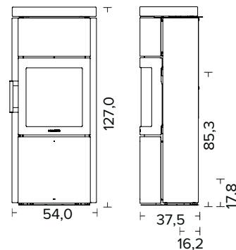
HWAM 3520c med fedtsten Standardgreb
