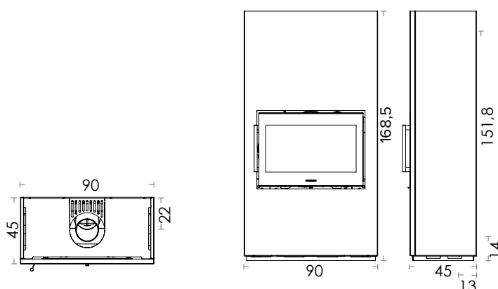
HWAM 5530c højrehængt låge
