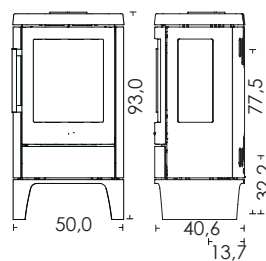
HWAM 4510c med lav sokkel HWAM® Autopilot™
