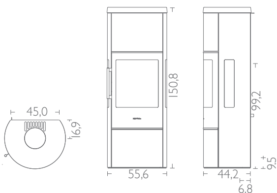
HWAM 3650c med sideglas
