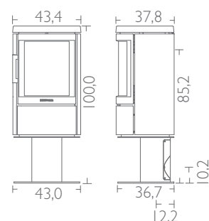
HWAM 2620c på piedestal
