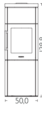
HWAM 4560m med fedtsten
