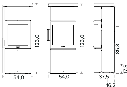
HWAM 3520c Style greb (rustfrit)
